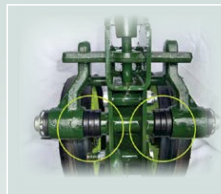
Arruelas de encosto, usadas para aproximar ou afastar o sistema de controle de profundidade em relação ao disco duplo da semente.
