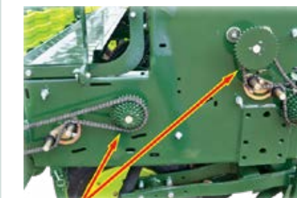
Sistema de Recâmbio, prático e versátil na regulagem da semente e adubo.
